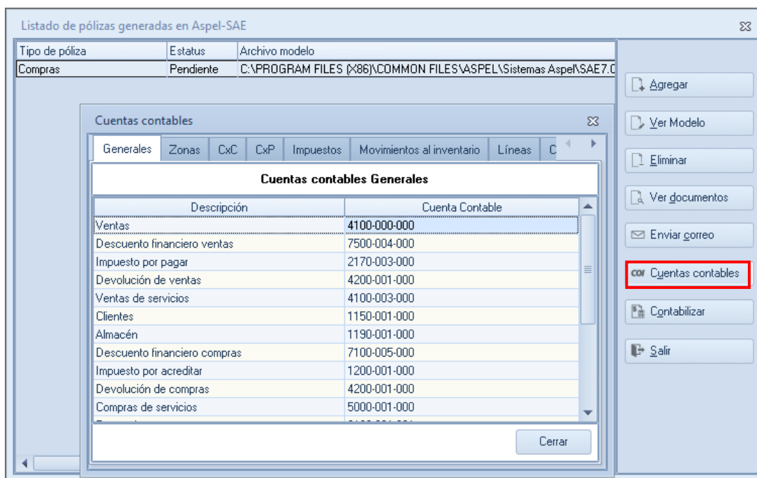
Configuración de las cuentas contables en los parámetros de la interfaz.
